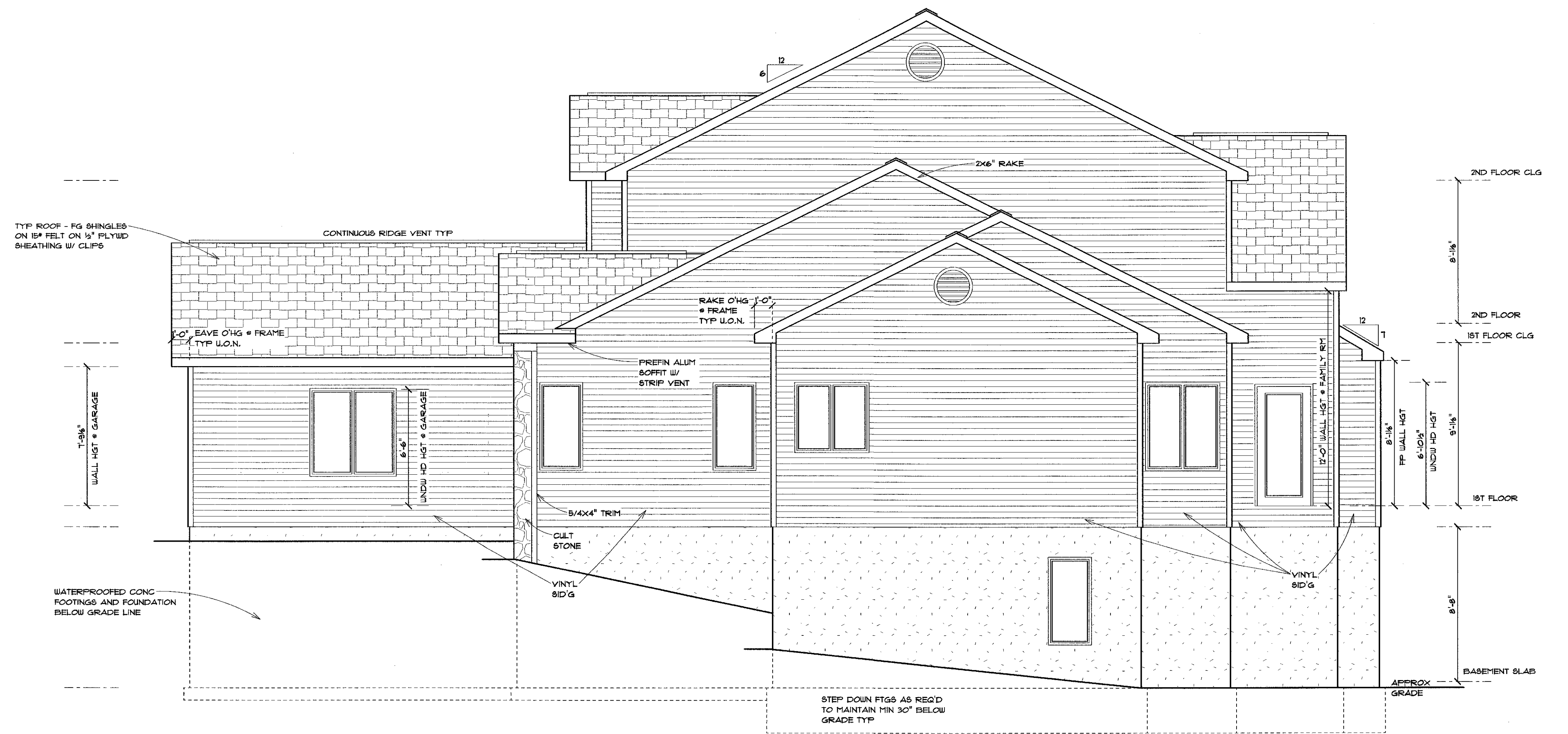
RIGHT ELEVATION
